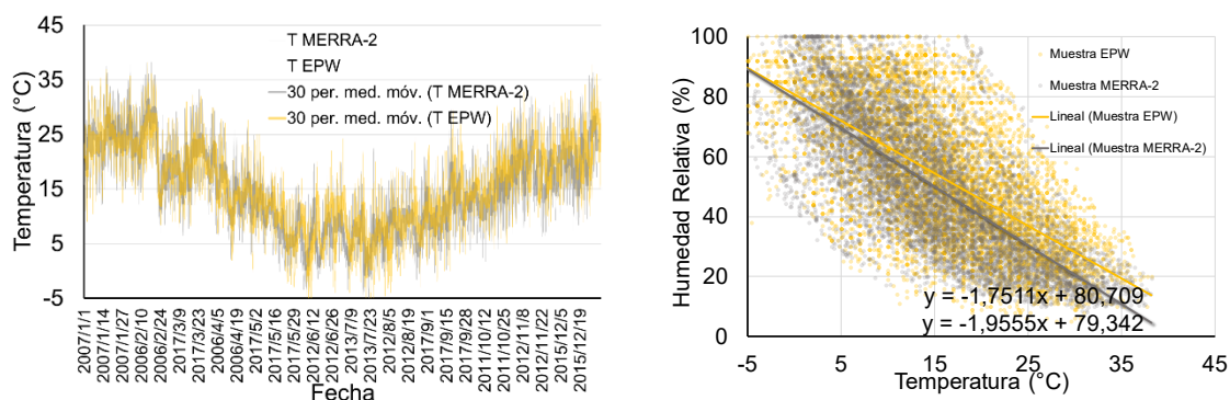
Figura 7. Neuquén. Comparación temperatura SMN y MERRA. A la izquierda, curva de T sobre eje temporal, y a la derecha diagrama de dispersión con línea de tendencia.
