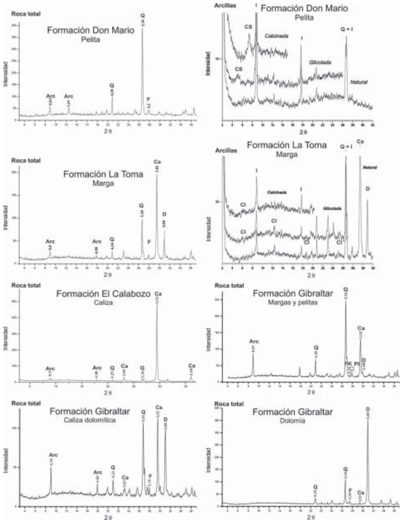
Figura 6. Difractogramas de rayos X (Arc: arcillas; Q: cuarzo; F: feldspatos; FK: feldespato potásico; Pl: plagioclasa; Ca: calcita; D: dolomita; I: illita; Cl: clorita; IS: interestratificado illita-esmecita; CS: interestratificado clotita-esmecita).
