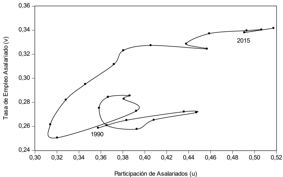
GRÁFICO 4.C: ESPACIO DE FASE (U,V) EN ARGENTINA: SUB-PERÍODO 1990-2015
