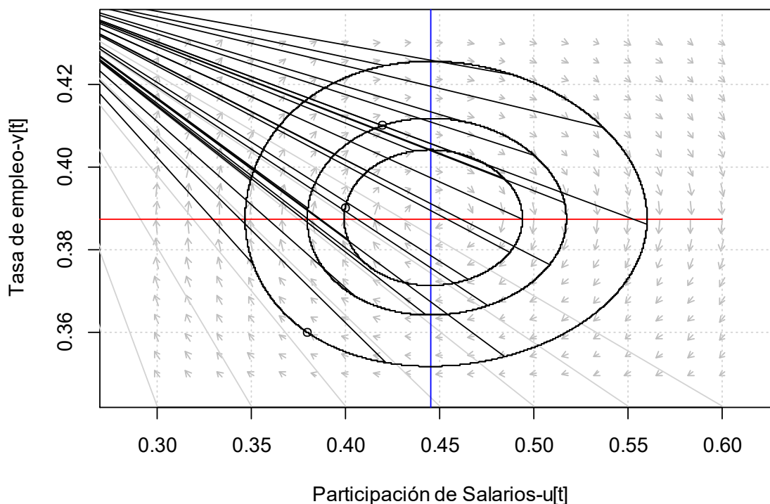
GRÁFICO 1: DIAGRAMA DE FASE TEÓRICO EN EL MODELO DE GOODWIN
