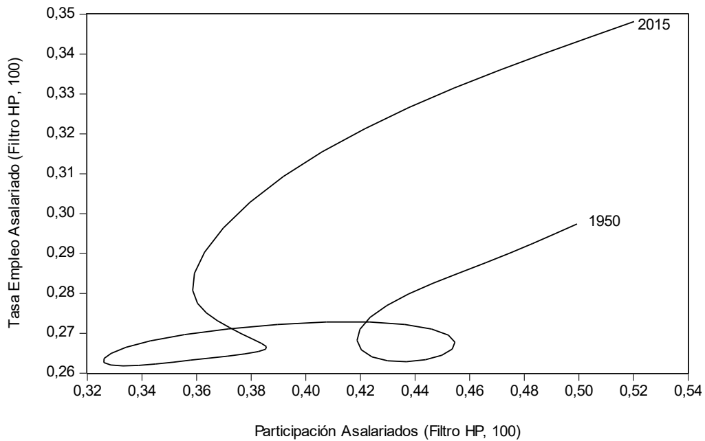
GRÁFICO 3: DIAGRAMA DE FASE: CICLOS DE LARGO PLAZO EN ARGENTINA (1950-2015)
