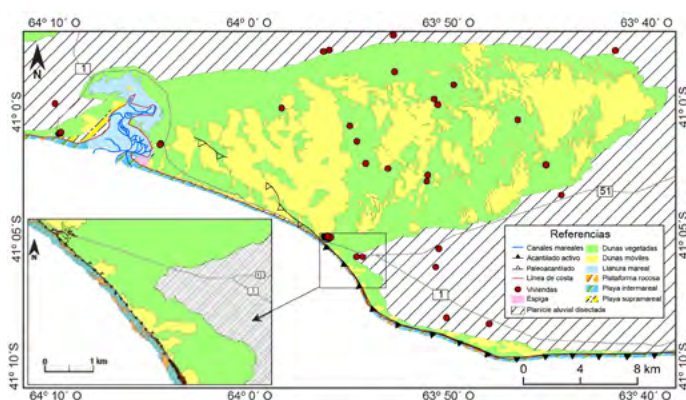
Figura 3. Mapa geomorfológico de la zona de estudio y alrededores. Tomado de Toffani (2018).
