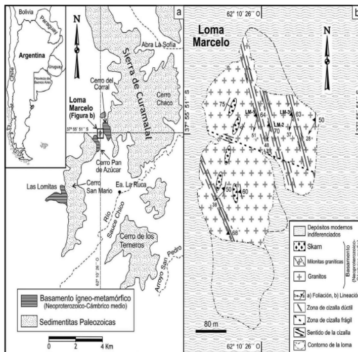
Figura 1. Mapa geológico del área en el que aflora el basamento proterozoico de las Sierras Australes (a) y detalle de la Loma Marcelo (b). Modificado de Lanfranchini et al. (2011).
